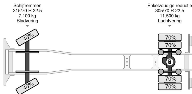
Volvo FL 240 EURO 5 EEV - 18 TON + DHOLLANDIA 4x2
