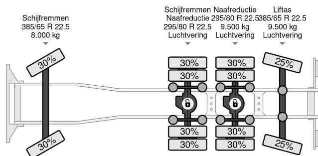
Mercedes-Benz Actros 2646 2646 8X4 HIAB 144E-4 HiPro +...
