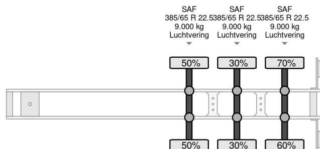
Kögel S***24 3x SAF BOX 1360x249x269
