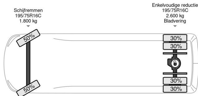
Iveco Daily 40 C17 + VELDHIJZEN 2019 YEAR!
