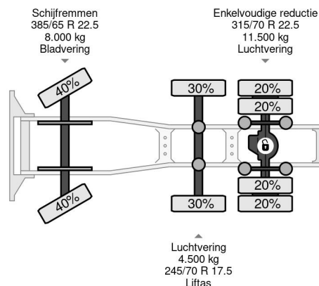
Volvo FH 500 6X2 EURO 6 DIESEL + LNG GAS
