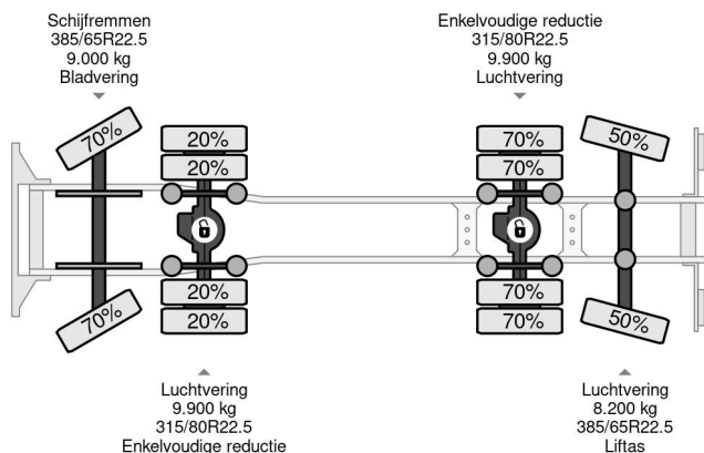
Scania P360 8X4 EURO 5 + HIAB 211 EP-4 + TIPPER
