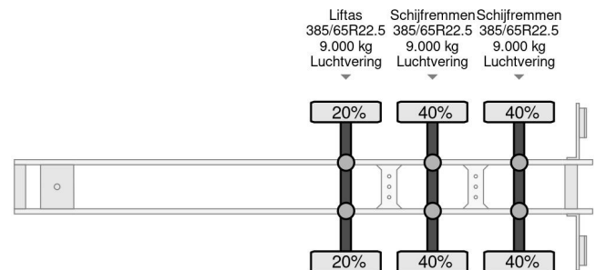
Benalu 3 AXLE - TIPPER - 24,9 M3
