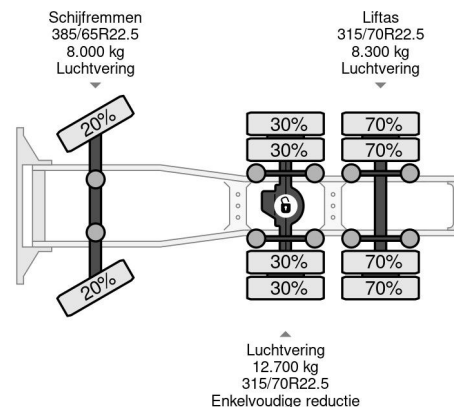
Scania T164-580 V8 6X2 + RETARDER + KIEPHYDRAULIEK...
