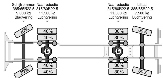
Volvo FMX 500 8X4 + HIAB 477 E-5 + JIB 100 X-4 + REMOT...
