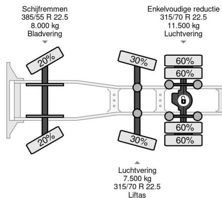
Volvo FH 460 6X2 EURO 6 i-Shift i-ParkCool
