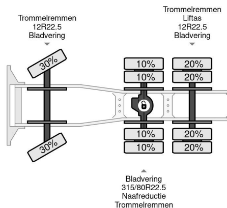
Volvo F 89 6X2 - F89TURBO6
