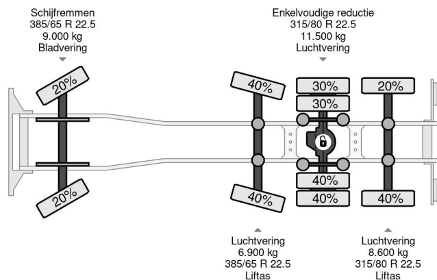
Scania R490 8X2 EURO 6 RETARDER
