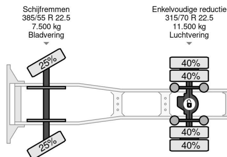
Scania R520 V8 NGS RETARDER + TUV 12/2024
