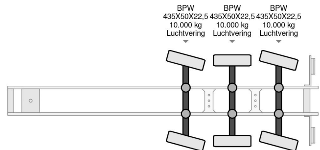
Renders 1 + 3e AXEL STEERING, LZV, 20,40,45 FT
