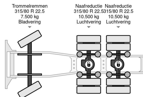
DAF CF 85.510 FTT 6X4 EURO 5 AUTOMATIC + ZF INTAR...
