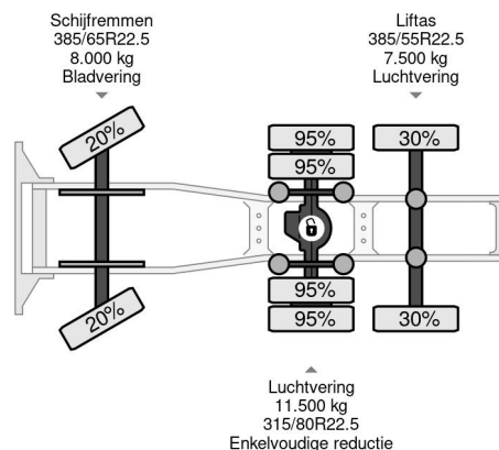
Volvo FH 500 6X2 EURO 5 + KIEPER HYDRAULIEK
