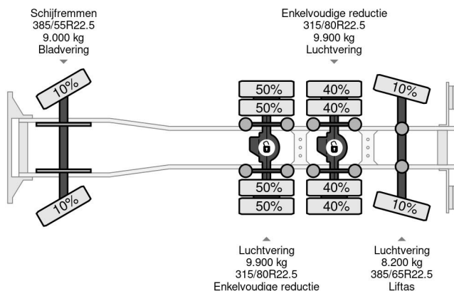
Scania P360 8X4 - EURO 5 + VDL 25T HOOK + TÜV 08-2025
