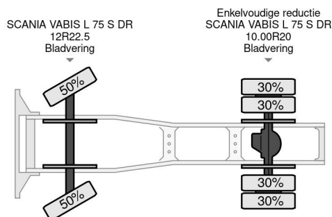
Scania L75 VABIS L 75 S DR 4X2
