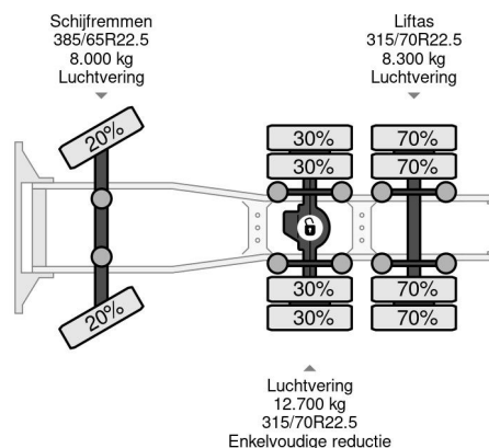
Scania T164-580 V8 6X2 + RETARDER + KIEPHYDRAULIEK...
