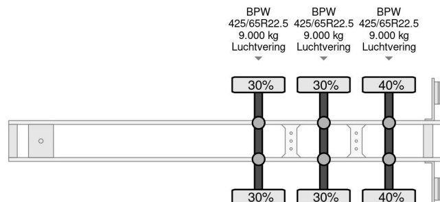
VAN HOOL 3C1017 - TIPPER - 56 M3 - STAHL/STEEL - 3 AX...
