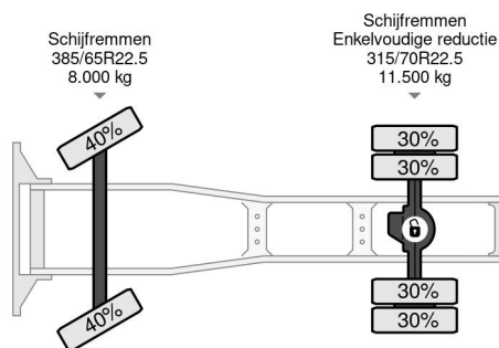
Scania R490 4X2 EURO 6 + RETARDER - APK 02/2025
