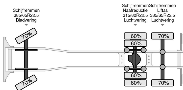
Renault T HIGH 520 6X2 EURO 6 + PALFINGER PK16002 R... Referentienummer: RE000746
