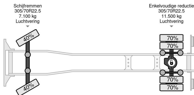
Volvo FL 250 4X2 EURO 6 CARGO LOCK + DHOLLANDIA L...
