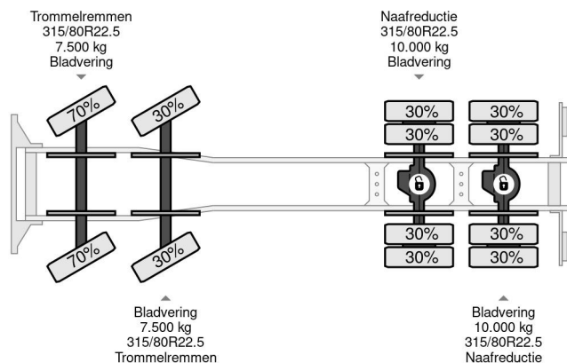
Volvo F 12 8X4 + CORMACH 87000 CRANE - 8.642 HOURS
