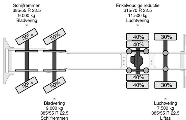
Volvo FMX 500 8X2 EURO 5 + HIAB 130 R F-1
