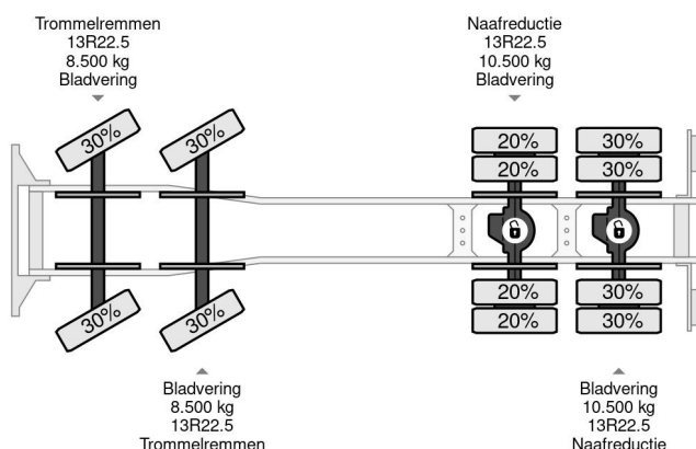
Scania P360 8X4 - EURO 5 + PALFINGER PK22002-EH + R...
