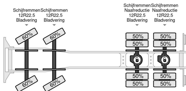
MAN TGS 35.400 8X4 PUTZMEISTER PUMP 21-3 + LIEBH...
