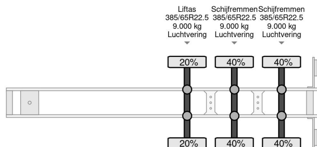
Benalu 3 AXLE - TIPPER - 24,9 M3
