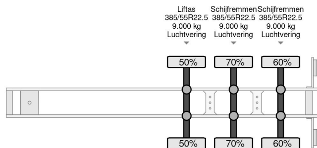
Hertoghs BOX TRAILER 3X SAF AXLE
