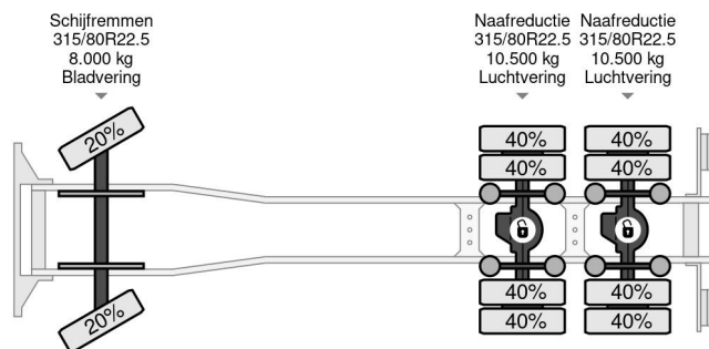
Iveco Stralis 450 6X4 - EURO 6 + MARREL 20T HOOK
