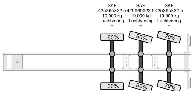
Floor 2 ASSEN GESTUURD
