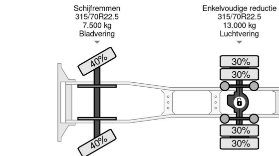
Mercedes-Benz Actros 1836 4X2 - EURO 6 + TÜV 09-2025
